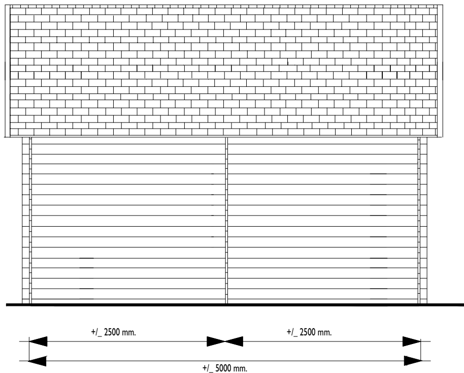
Zij aanzicht Seiten Ansicht Side view
