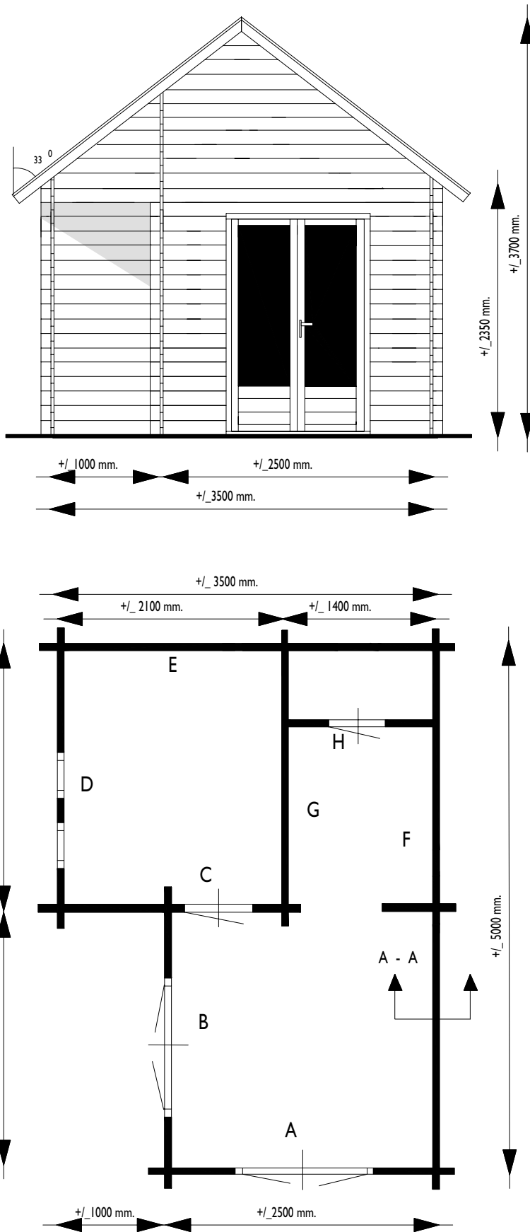
Voor aanzicht Vorder Ansicht Front view
